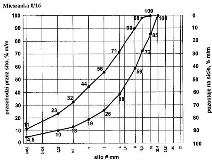
Rys.3. Uziarnienie mieszanki CBGM 0/16
