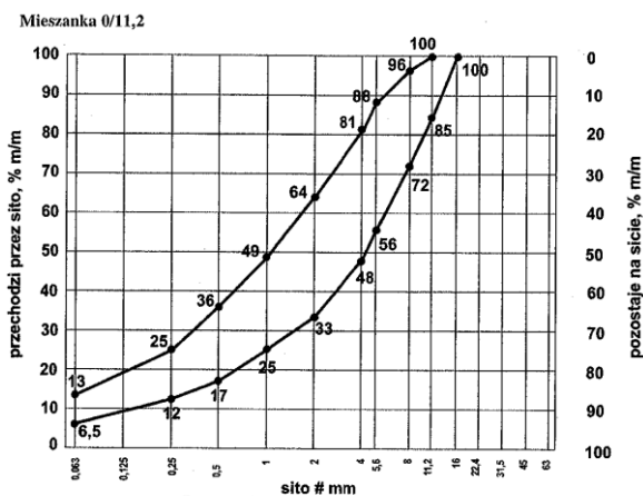
Rys.4. Uziarnienie mieszanki CBGM 0/11,2
