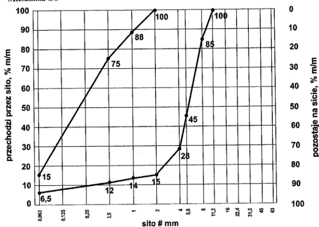
Rys.5. Uziarnienie mieszanki CBGM 0/8
